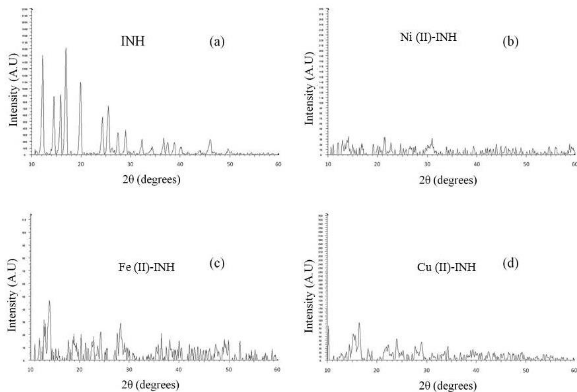
Fig. 2: X-ray diffractograms of (a) pure Isoniazid (INH), (b) Ni(II)-INH, (c) Fe(II)-INH and (d) Cu(II)-INH complexes.
